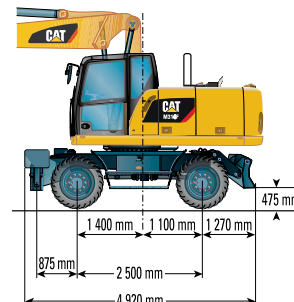
Podvozek s jednou soupravou opěrných noh a radlicí
