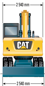
Podvozek pouze s radlicí
