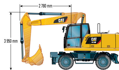
Podvozek s jednou soupravou opěrných noh a radlicí
